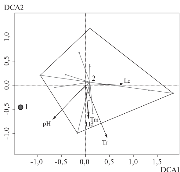
Рис. 3. DCA-ординація угруповання за участю Allium ursinum і Euonymus nana (синтаксон 1) та інших угруповань лісової рослинності (синтаксон 2) Національного дендрологічного парку «Софіївка» НАН України
