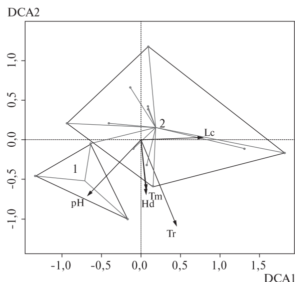
Рис. 4. DCA-ординація угруповання за участю Scopolia carniolica (синтаксон 1) та інших угруповань лісової рослинності (синтаксон 2) Національного дендрологічного парку «Софіївка» НАН України
