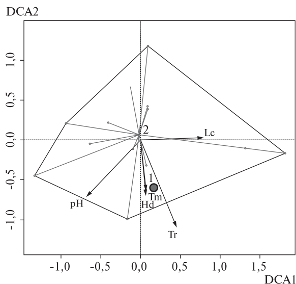
Рис. 2. DCA-ординаяція угруповання за участю Tulipa quercetorum (синтаксон 1) та інших угруповань лісової рослинності (синтаксон 2) Національного дендрологічного парку «Софіївка» НАН України. Тут і на рис. 3 і 4: Lc — освітлення; Tm — терморегімі; Hd — вологість; pH — реакція ґрунту; Tr — вміст поживних речовин у ґрунті
