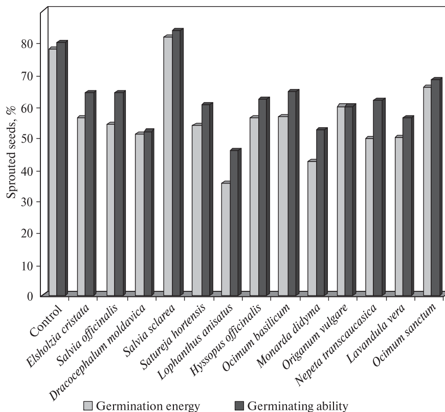
Рис. 4. Алелопатичний вплив водних екстрактів післяжнивних решток ароматичних рослин на проростання насіння кукурудзи (середні дані за 2010–2012 рр.)
